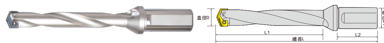
SD spade drill (槽型辨别: H型 螺旋槽 S型 直行槽)
