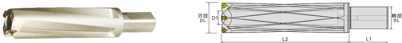
AMD nesting drill (系列辨别: AMD10即 10系列)
