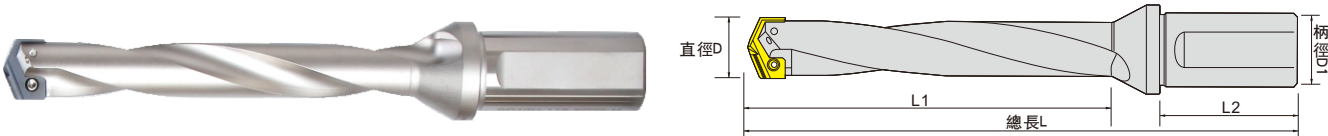
SD spade drill (槽型辨别: H型 螺旋槽 S型 直行槽)
